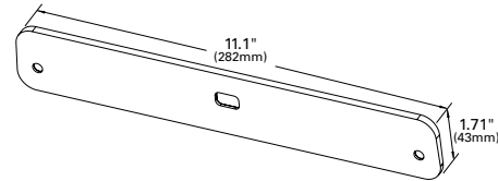
Gasket
