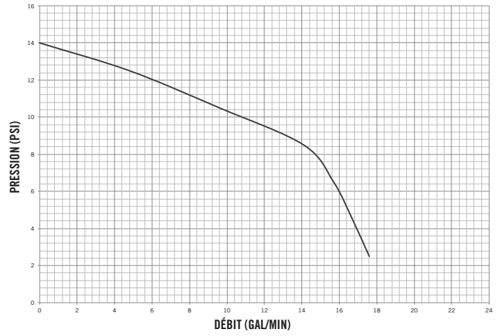
COURBE CARACTÉRISTIQUE : SÉRIE 2400 (24 VCC)
