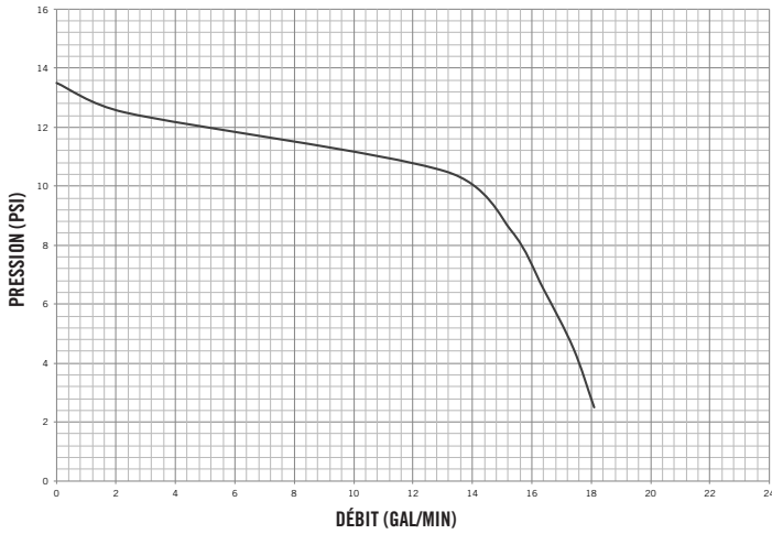
COURBE CARACTÉRISTIQUE : SÉRIE 1200 (12 VCC)
