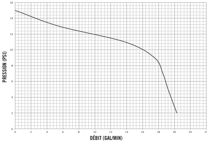
COURBE CARACTÉRISTIQUE : SÉRIE 4200 (12 VCC)
