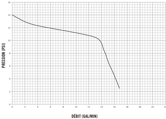
COURBE CARACTÉRISTIQUE : SÉRIE 600 (115 VCA)
