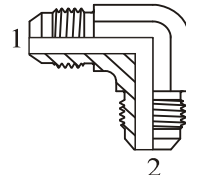
MJ X MJ 90°
